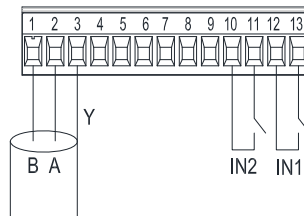
Figura 7: Morsettiere estraibile 13 poli: ingressi digitali e MODBUS
